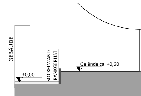
SCHEMA - SCHNITT
